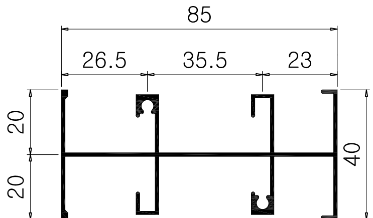
KAT85SL-305 0.93 kg/m 1.0 T
