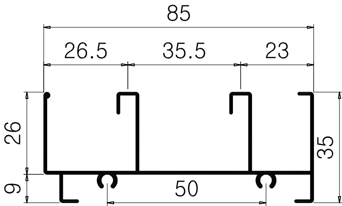
KAT85SL-102 0.72 kg/m 1.0 T
