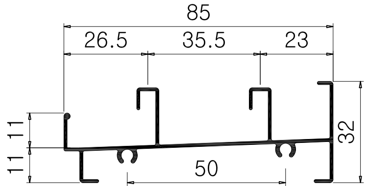
KAT85SL-204 0.64 kg/m 1.0 T
