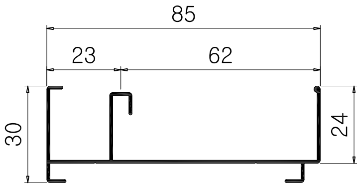
KAT85SL-304 0.52 kg/m 1.0 T
