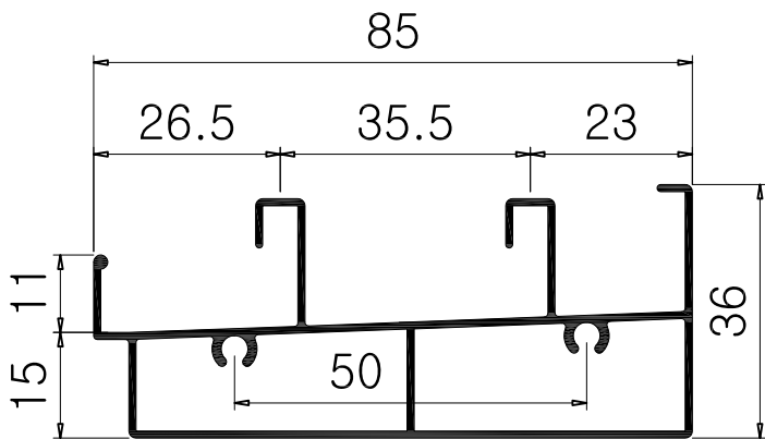
KAT85SL-206 0.85 kg/m 1.0 T
